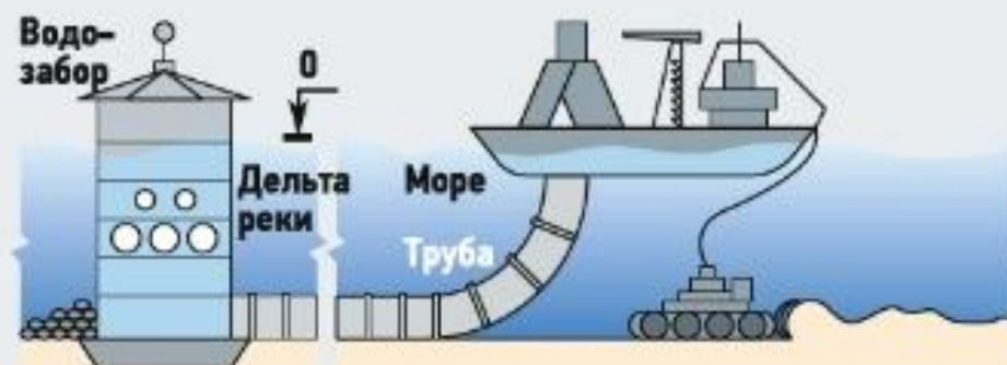
Эластичный водовод (диаметром до 3 м)
